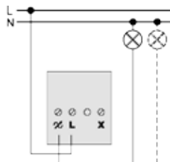
Поворотний світлорегулятор MTN5131-0000.
