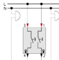
2-кнопковий вимикач, 2 замикаючих контакти MTN3155-0000
