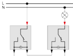
Перемикач з підсвічуванням MTN3136-0000
