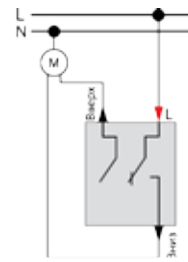
Клавішний вимикач для жалюзі, 1-полюсний MTN3715-0000
