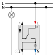
Перемикач з контрольною лампою MTN3106-0000
