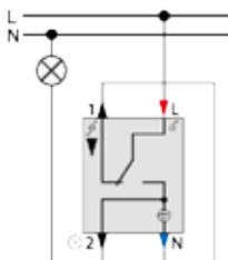
Перемикач з контрольною лампою MTN3106-0000
