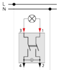
Двополюсний вимикач на один напрямок з контрольною лампою MTN3102-0000
