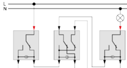
Перемикач з підсвічуванням MTN3136-0000
