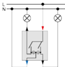
2-клавiшний вимикач з контрольною лампою MTN3105-0000
