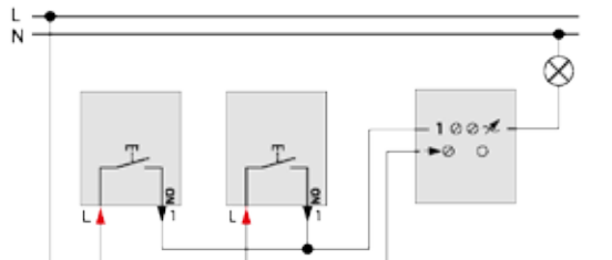
Кноповий вимикач як основний пристрій.
