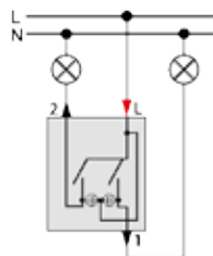
2-клавiшний вимикач з підсвічуванням MTN3135-0000
