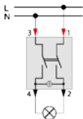
Двополюсний вимикач на один напрямок з контрольною лампою MTN3102-0000
