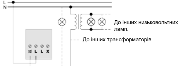
Поворотний світлорегулятор MTN5133-000.
