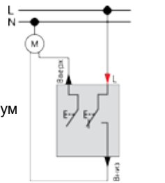
Кнопковий вимикач для жалюзі, 1-полюсний MTN3755-0000
