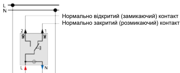
Кнопковий перемикач із клемою нейтралі MTN3156-0000 Світлодіодний модуль підсвічування для клавішних/кнопкових вимикачів MTN3901-00**, MTN3921-0000
